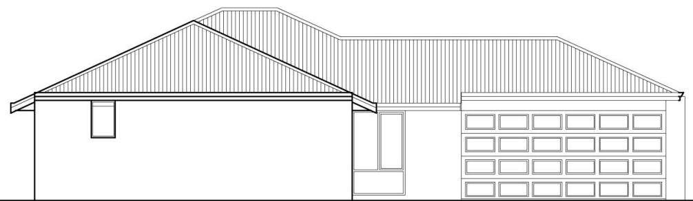
ELEVATION B
